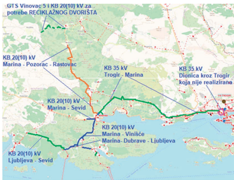
Slika 1 - Stanje i poboljšanja elektroenergetske mreže na području Općine Marina
