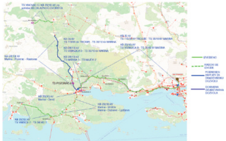
Slika 1 – Stanje i poboljšanja elektroenergetske mreže na području općine Marina
