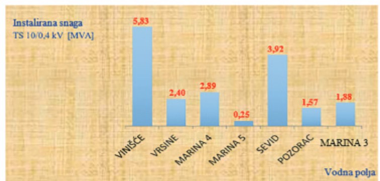
Slika 2 – Instalirana snaga TS 10/0,4 kV na području općine Marina po vodnim poljima 10 kV iz TS 35/10 kV Marina
